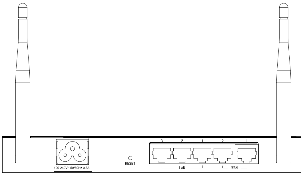
图 2-4 TL-WVR300后面板示意图
