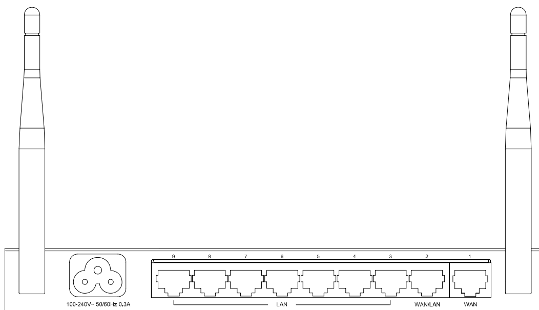
图 2-6 TL-WVR308后面板示意图
